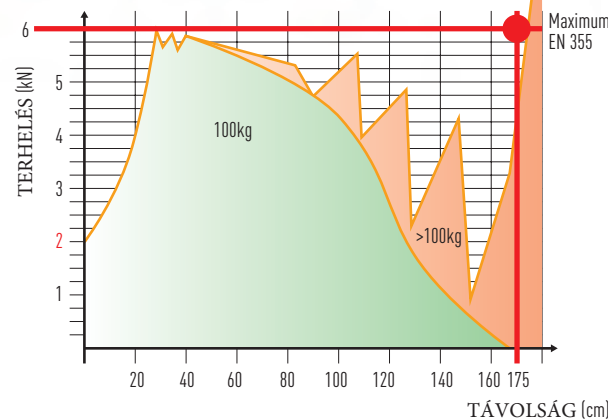
A HAGYOMÁNYOS ENERGIAELNYELŐK SÜLYKOMPENZÁLÁSI KINYÚLÁSA
