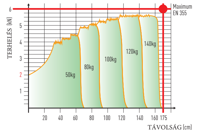
AZ ONE4ALL ENERGIAELNYELŐ SÜLYKOMPENZÁLÁSI KINYÚLÁSA
